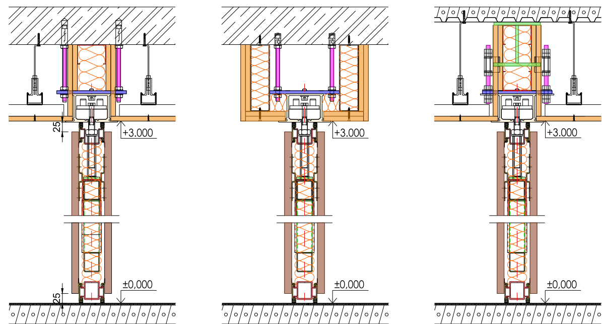
Vertikální řezy kotvením stěnou Palace:
