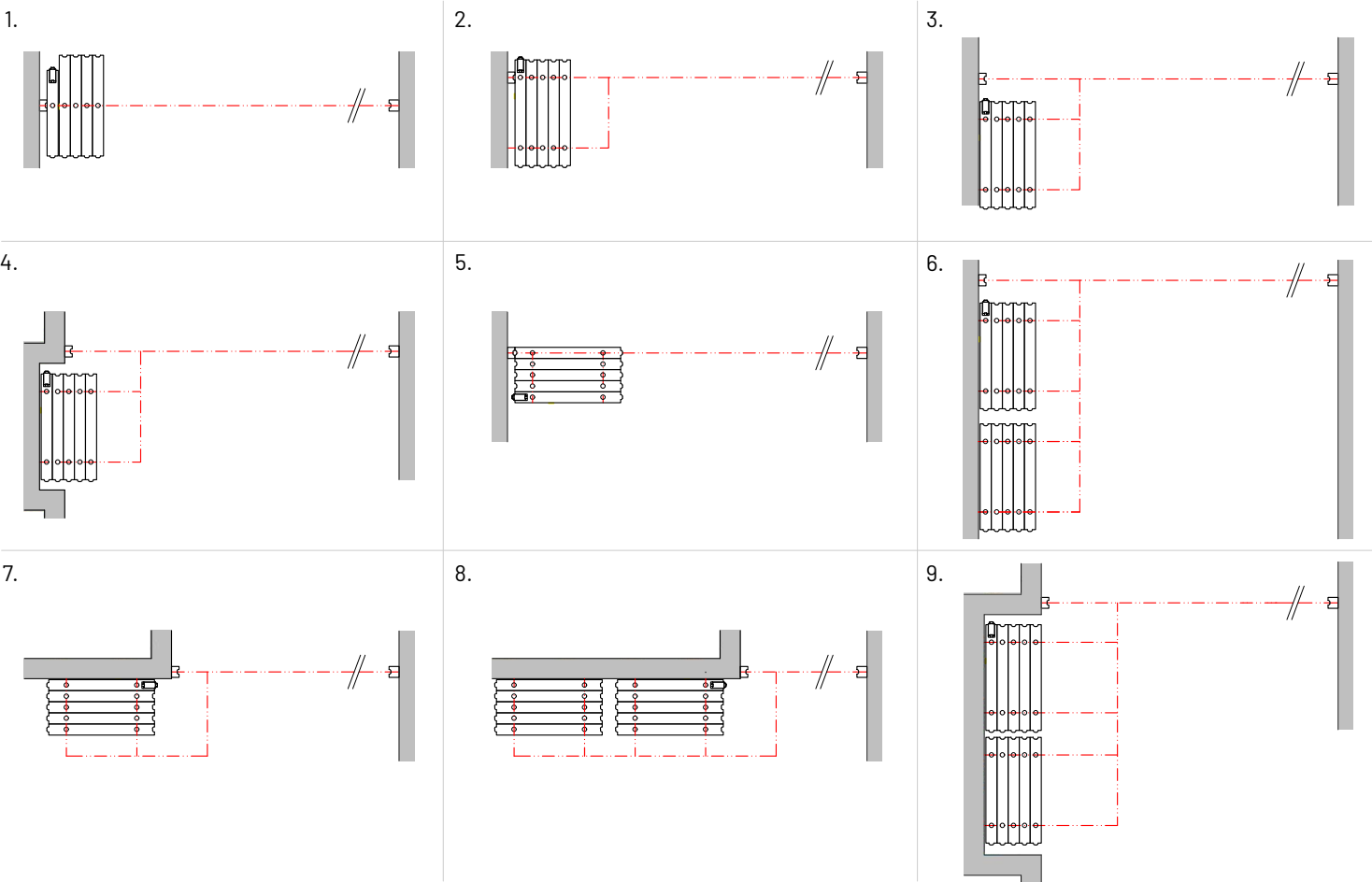
1: Jednobodové zavěšení
