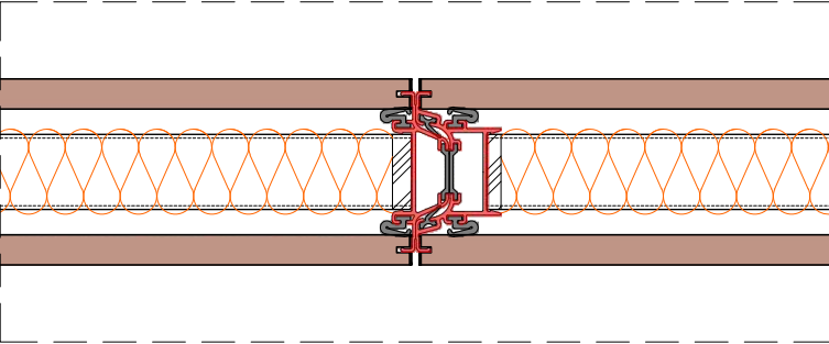
Horizontální řez:
