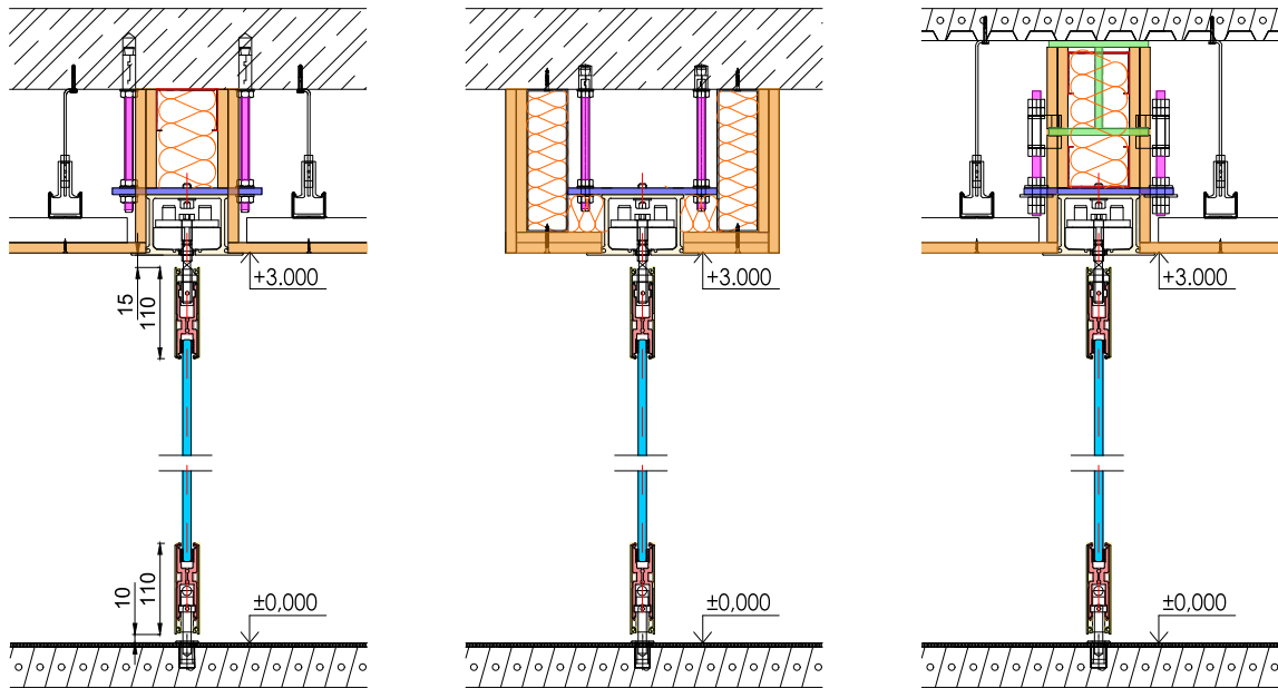
Vertikální řezy kotvením stěnou President:
