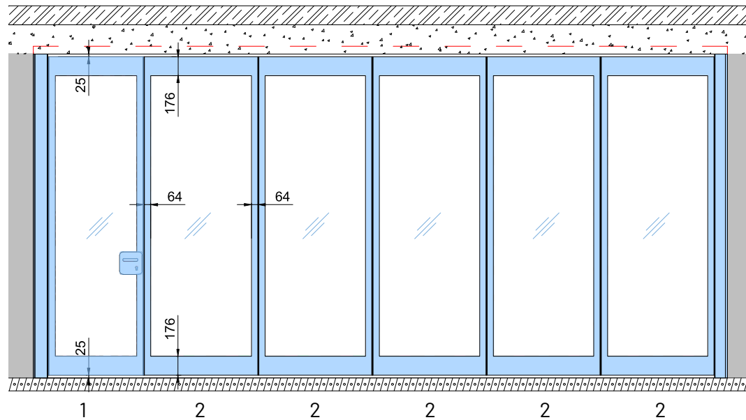
Stěna zavřená:
