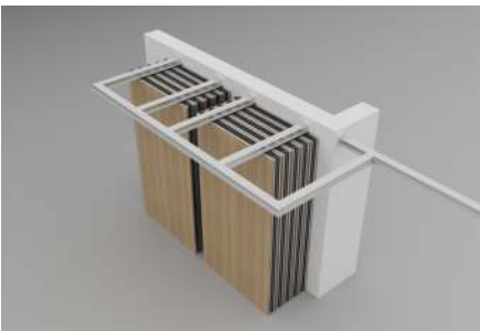
8: Dvoubodové zavěšení
