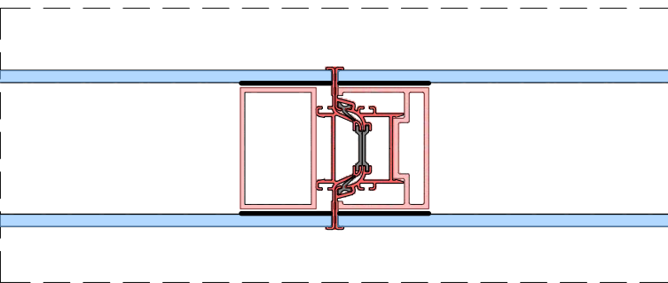
Horizontální řez:
