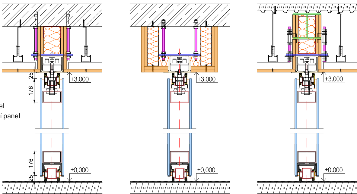
Vertikální řezy kotvením stěnou Palace Glass Premium:
