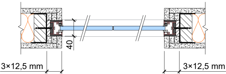
Horizontálny rez
