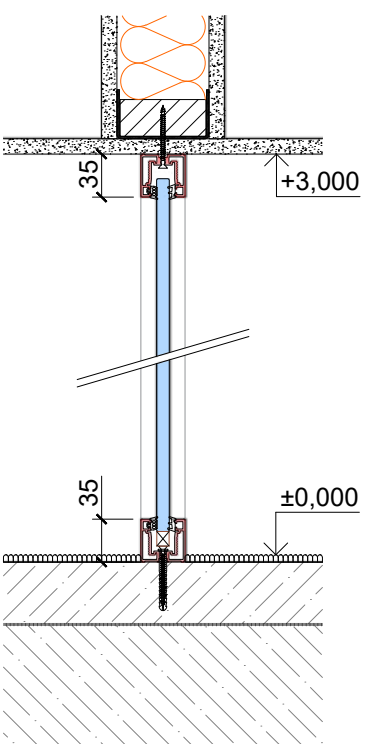
Vertikálny rez
