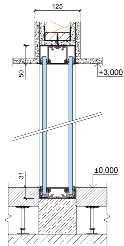
Vertikálny rez
