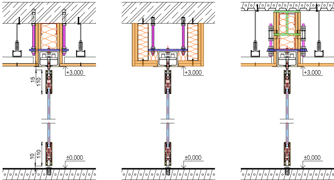
Vertikálne rezy kotvením stenou President:
