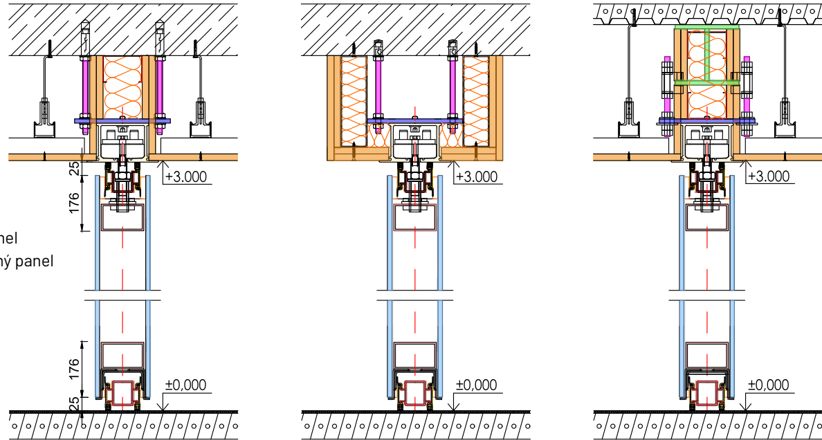
Vertikálne rezy kotvením stenou Palace Glass Premium:
