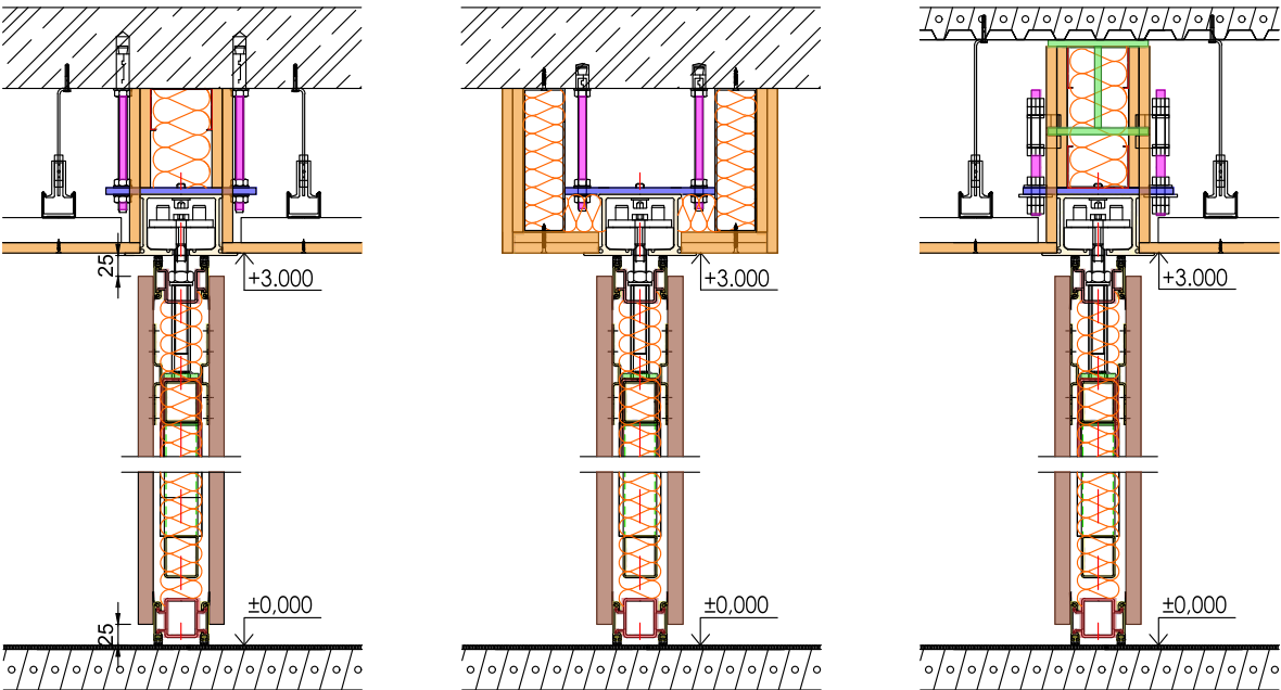
Vertikálne rezy kotvením stenou Palace:
